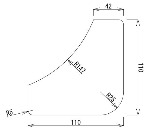
コーナー用ゴムクッション 拡大図
